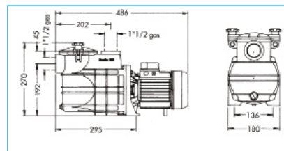
Afmetingen in mm
